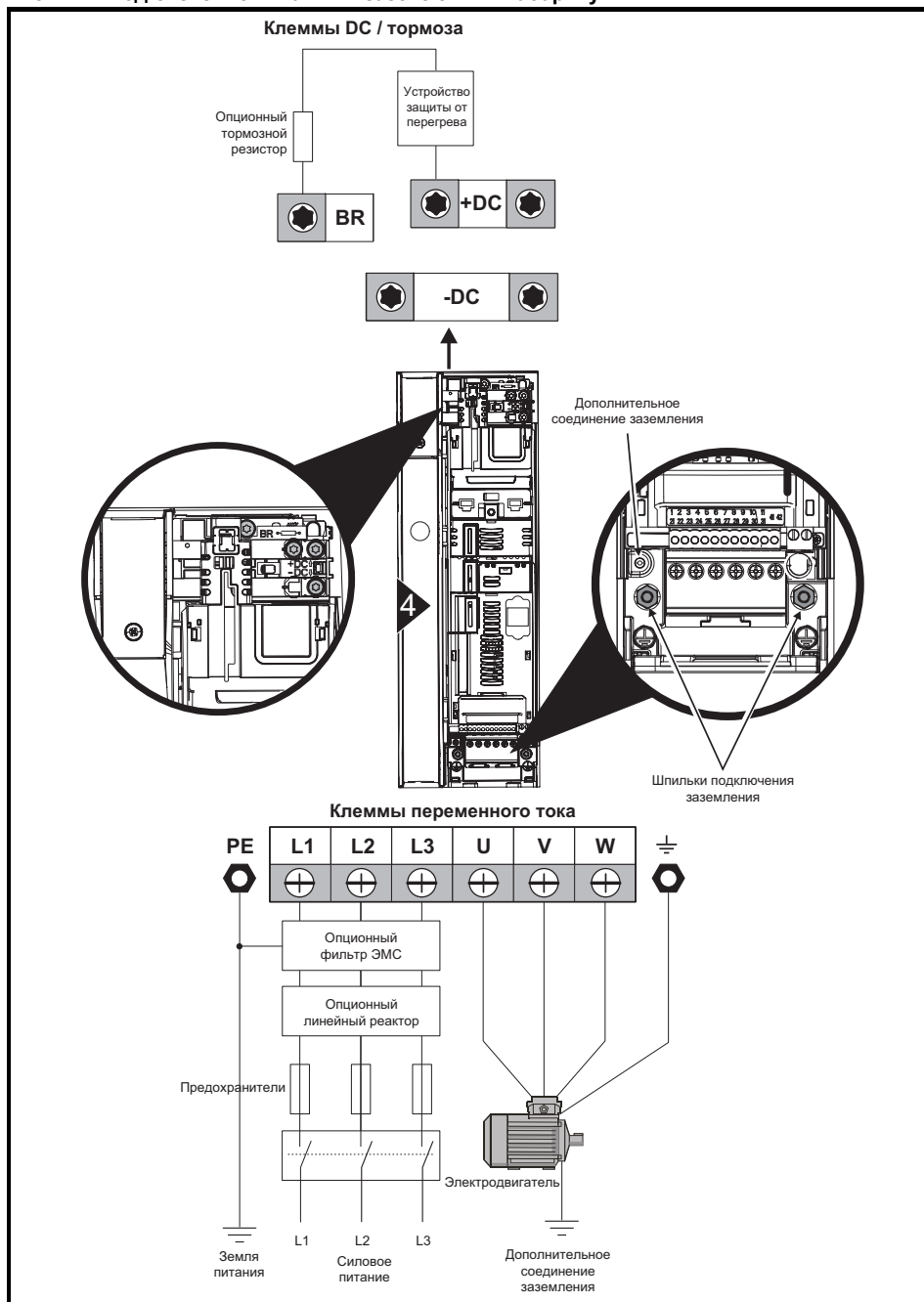
Рис. 4-2 Подключение питания и заземления к габариту 4
